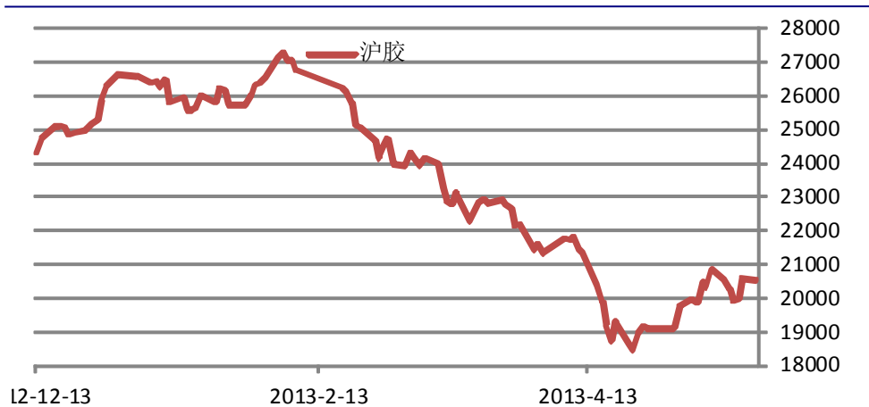
图 1: 沪胶走势图
